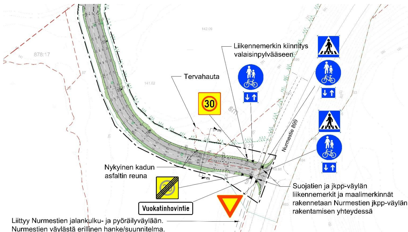
Kuva 8. Vuokatinhovintien katusuunnitelma Nurmestien liittymän kohdalta.
